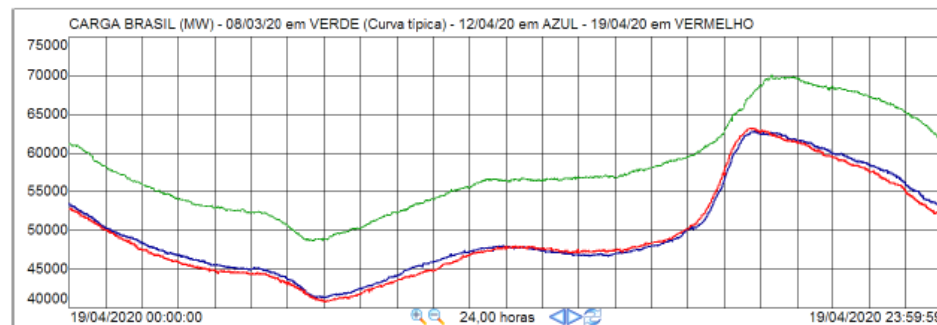
CURVA DE CARGA DO SIN (CURVA TÍPICA X VERIFICADO X SEMANA ANTERIOR)
